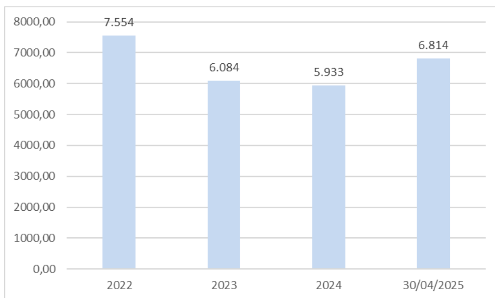
Figura 3. Indice di consumo di metano ( Sm^3/M euro).
